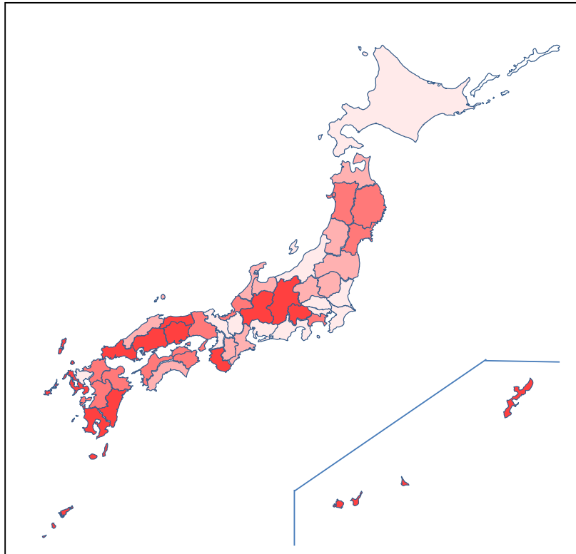
土砂災害
